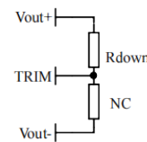
电压下调: 在Trim和输出正之间增加电阻Rdown Rdown = 15 * (15 - 2.5 - \Delta U) / \Delta U - 5.1 (K \Omega )
