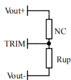
电压上调: 在Trim和输出负之间增加电阻Rup Rup = 37.5 / \Delta U - 5.1 (K \Omega )
